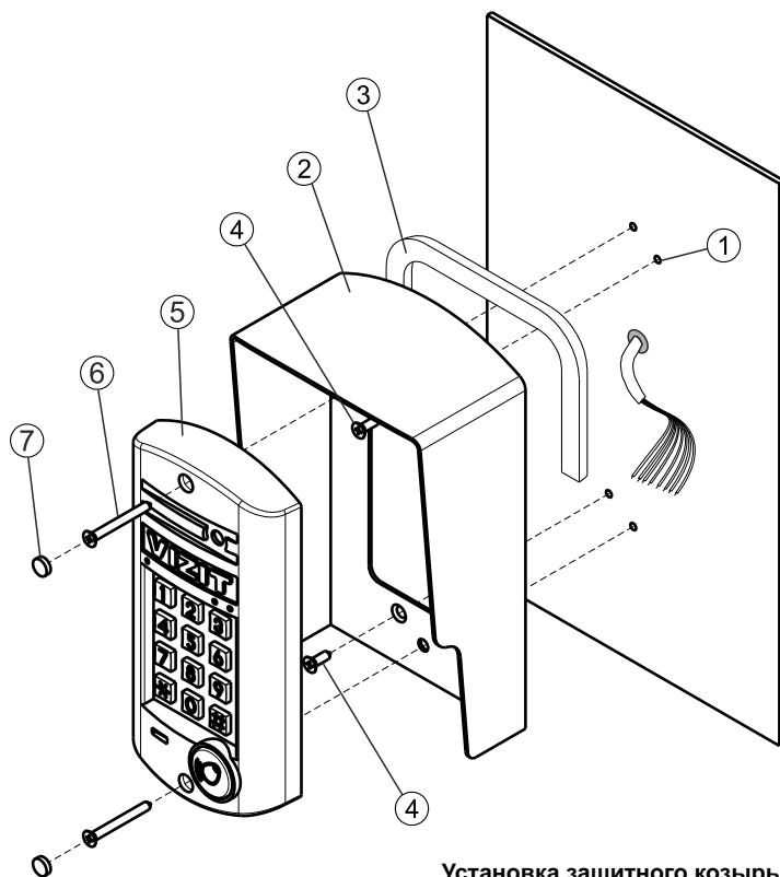
Установка защитного козырька и накладного блока БВД-312х (-313х, -314х, -315х, -343х, -344х) на металлическую дверь
