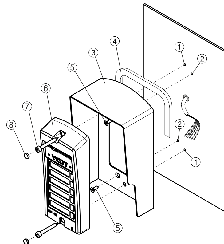
Установка защитного козырька и накладного блока БВД-306х (-310х, -316х, -SM110х) на металлическую дверь
