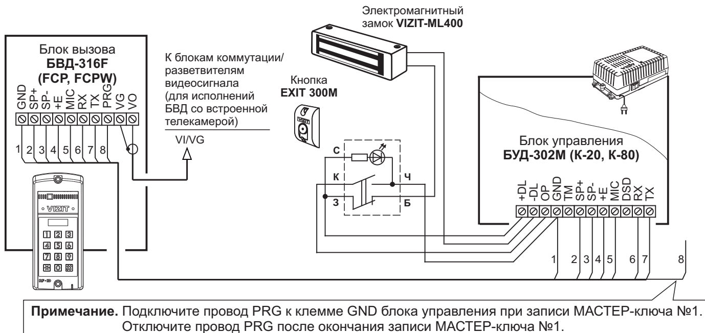
Рисунок 6 - Схема соединений блока вызова БВД-316F(FCP, FCPW) с блоком управления БУД-302M (K-20, K-80) , электромагнитным замком VIZIT-ML400 и кнопкой EXIT 300M
