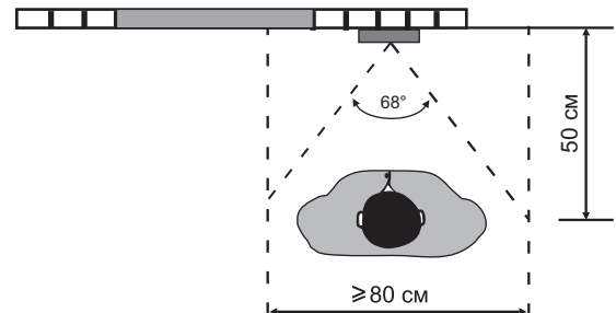
Рисунок 4 - Рекомендуемая высота установки блока вызова и область обзора телекамеры
