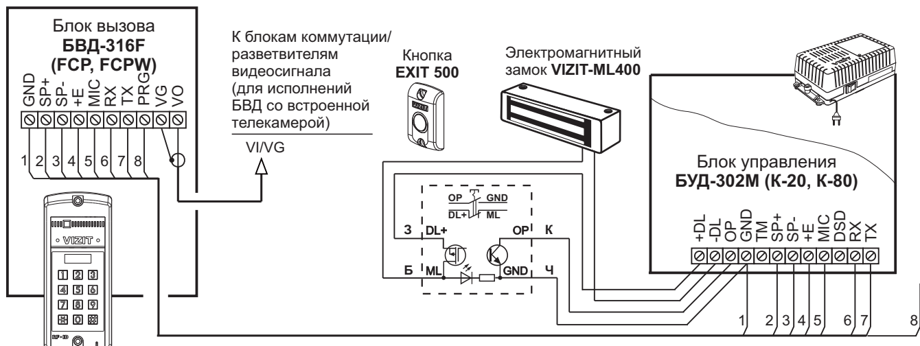
Рисунок 7 - Схема соединений блока вызова БВД-316F(FCP, FCPW) с блоком управления БУД-302M (K-20, K-80) , электромагнитным замком VIZIT-ML400 и кнопкой EXIT 500
