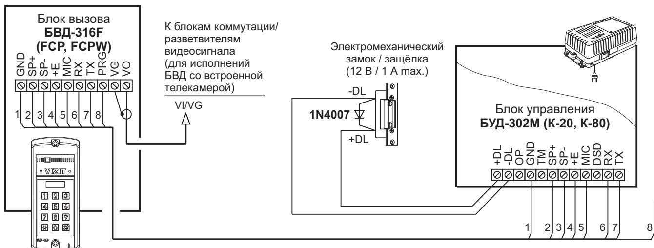
Рисунок 7 - Схема соединений блока вызова БВД-316F(FCP, FCPW) с блоком управления БУД-302M (K-20, K-80) , электромагнитным замком VIZIT-ML400 и кнопкой EXIT 500
