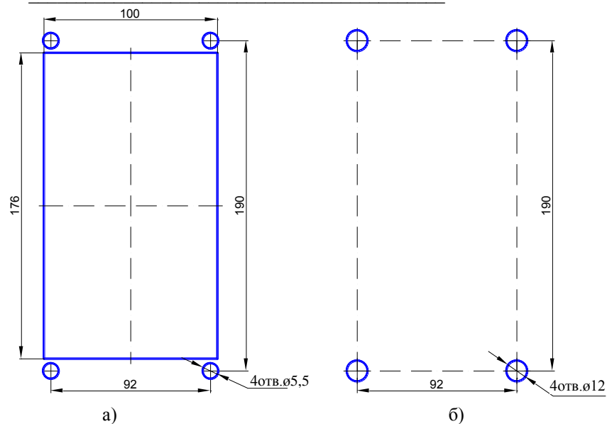
Рис1. Разметка под крепление DP400-RDC24 а) снаружи; б) изнутри.
