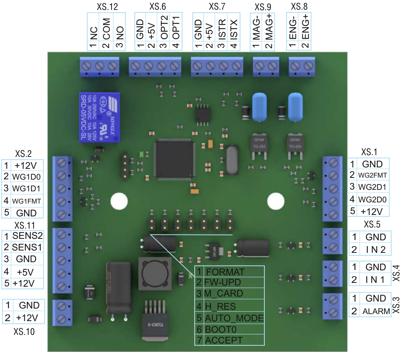
Рисунок 2.1 Контроллер управления турникетом «СВU-260»
